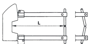
Typ 7501 L = 125 mm Typ 7502 L = 250 mm Typ 7503 L = 350 mm Typ 7504 L = 500 mm Typ 7521 Ø 10 ▲
