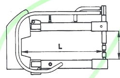
Typ 7512 L = 150 mm Typ 7513 L = 250 mm Typ 7514 L = 350 mm Typ 7515 L = 500 mm Typ 3830 ▲
