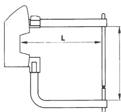
Typ 7506 L = 250 mm Typ 7511 L = 125 mm Typ 7523 Ø 10 ▲
