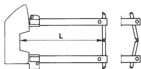
Typ 7401 L = 125 mm Typ 7402 L = 250 mm Typ 7403 L = 350 mm Typ 7404 L = 500 mm Typ 7451 Ø 12 ▲
