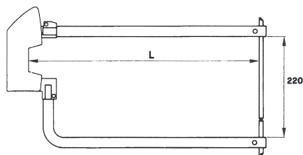
Typ 7406 L = 350 mm Typ 7407 L = 500 mm Typ 7453 Ø 12 elektrodo inferiore/lower electrode /électrode inférieure Typ 7454 Ø 12 elektrodo superiore/upper electrode /électrode supérieure
